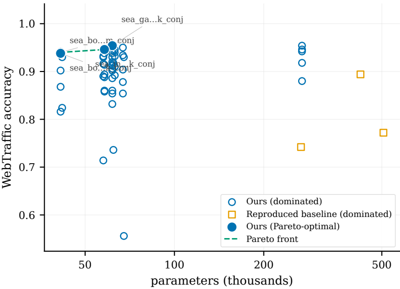
Accuracy vs Parameters
