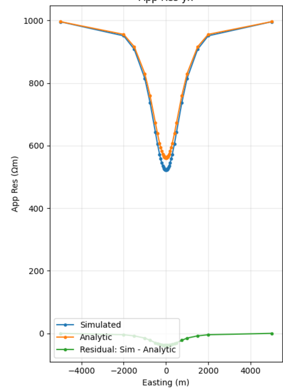
App Res yx
