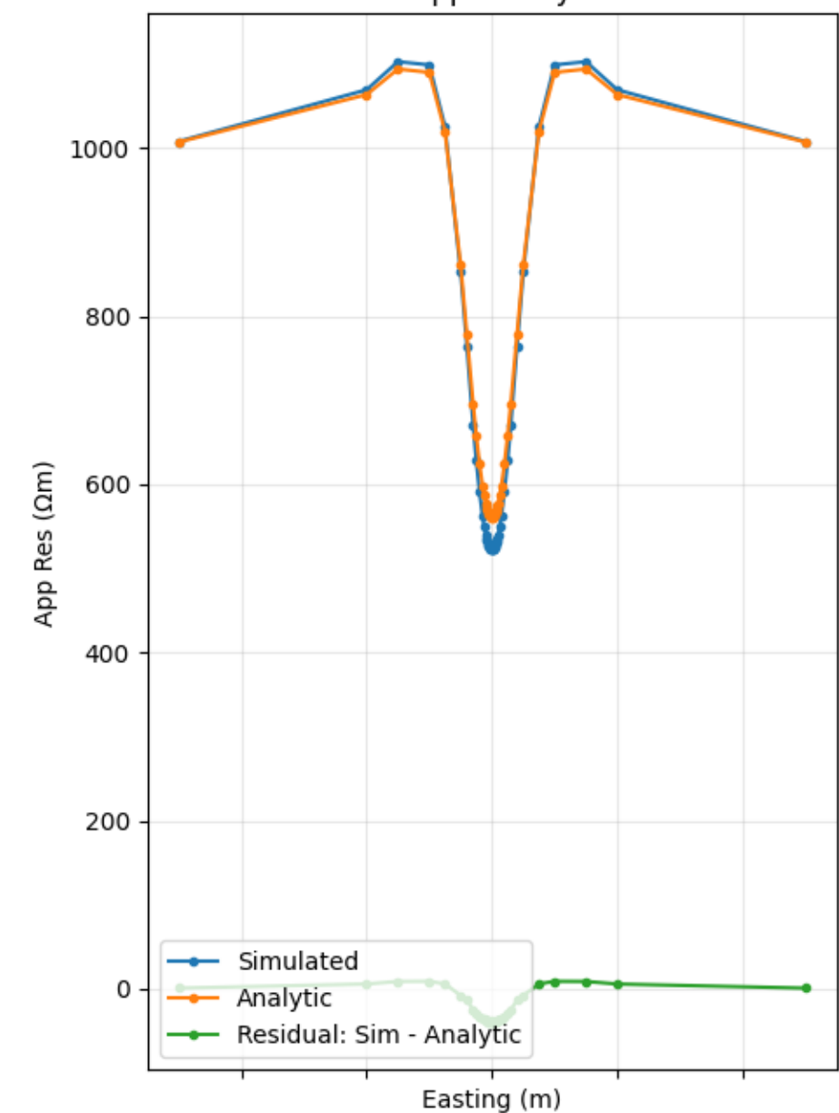
App Res yx
