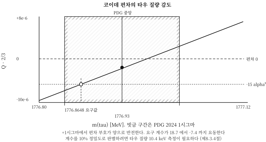
Figure 4. 코이데 편차의 타우 질량 감도 - PDG 2024 1\sigma 구간 안에서 편차의 값과 부호가 판별 불가 구간을 지난다.
