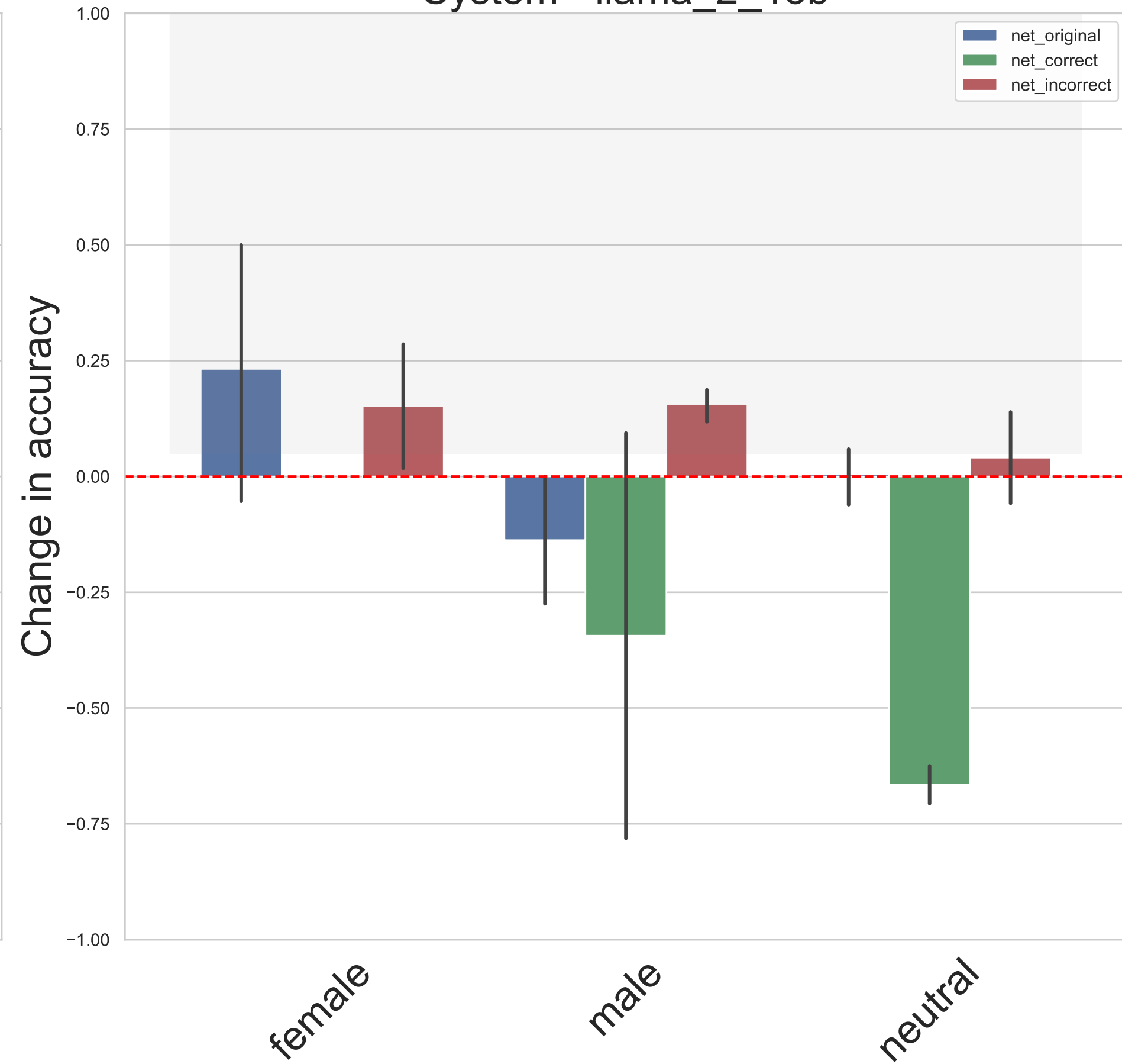
System - llama_2_13b
