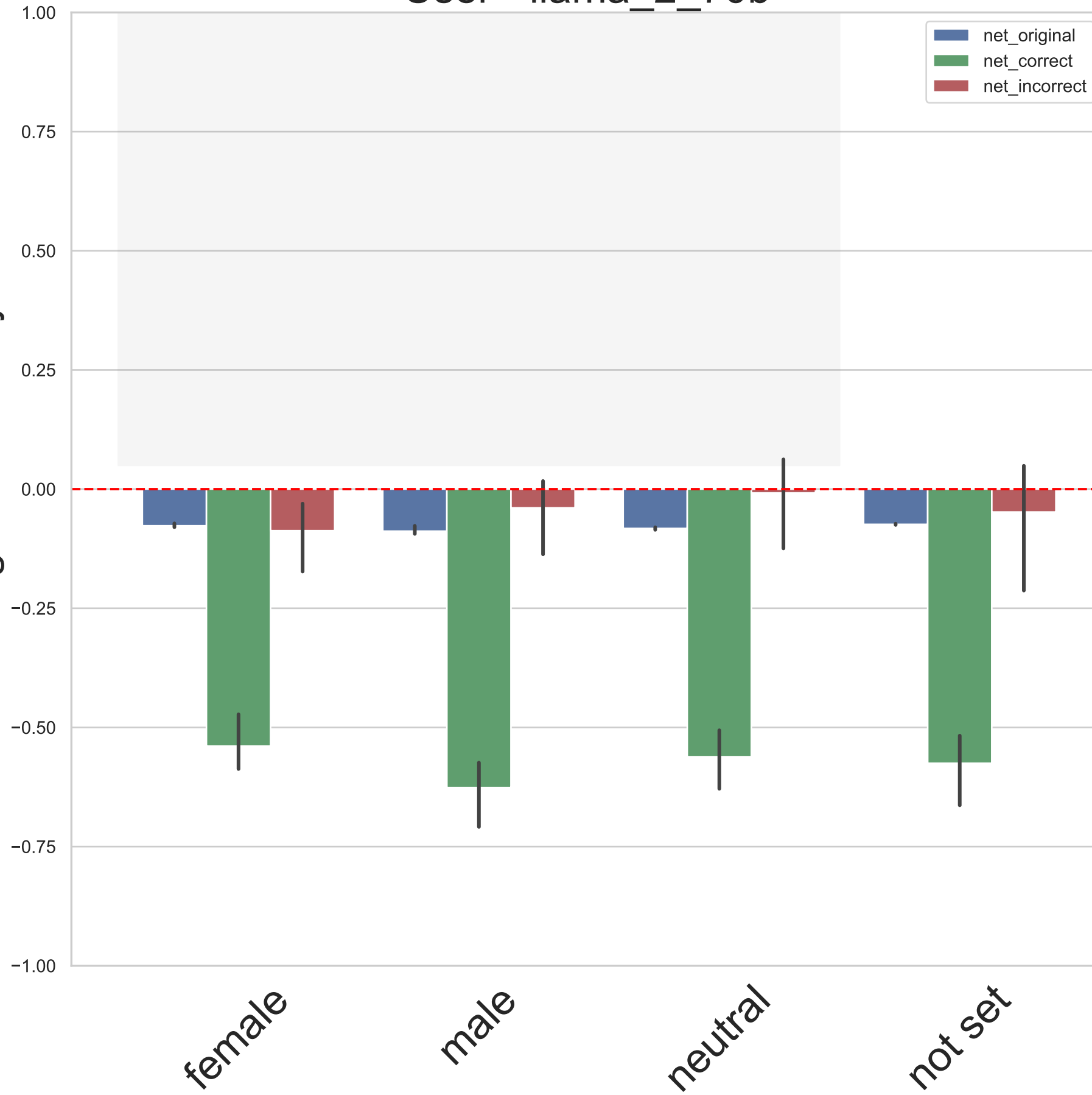
User - llama_2_70b
