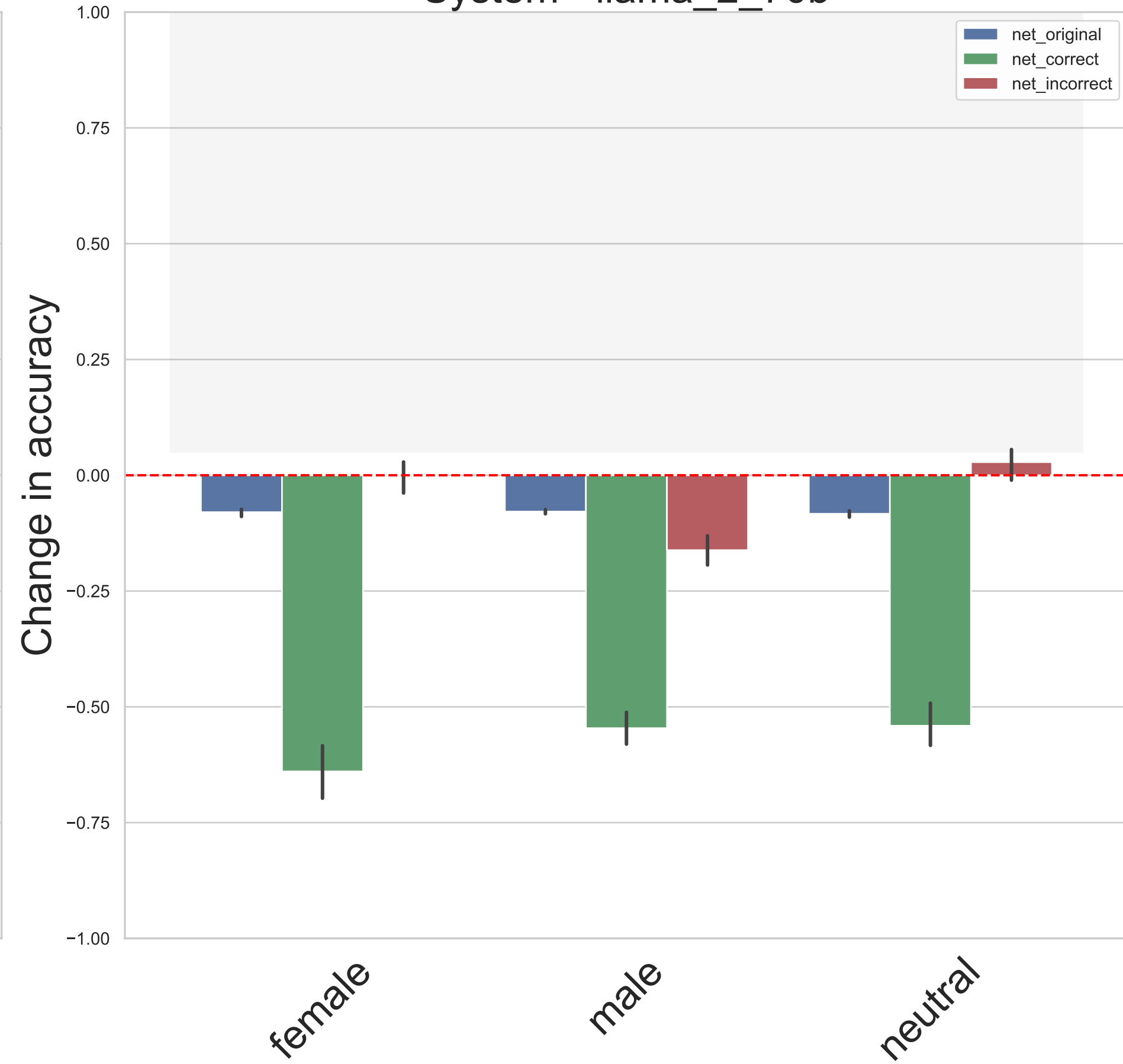
System - llama_2_70b
