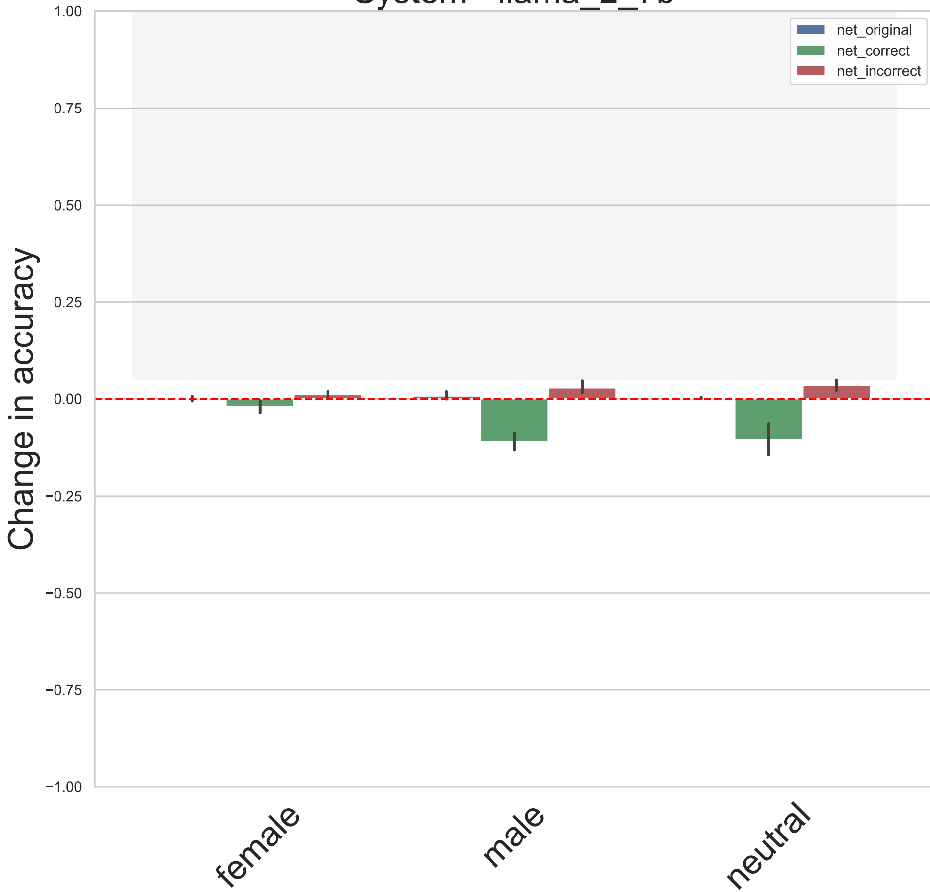
System - llama_2_7b
