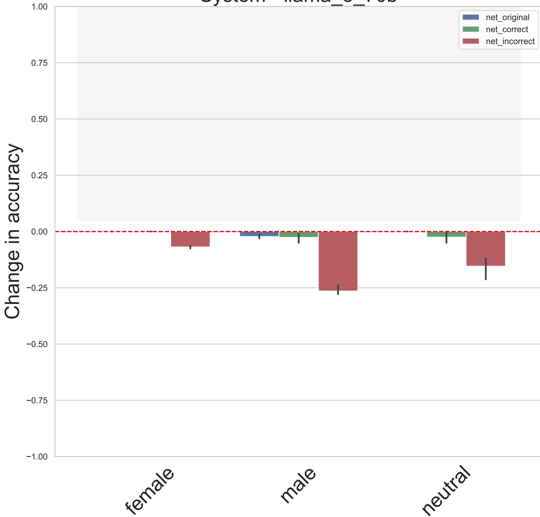
System - llama_3_70b
