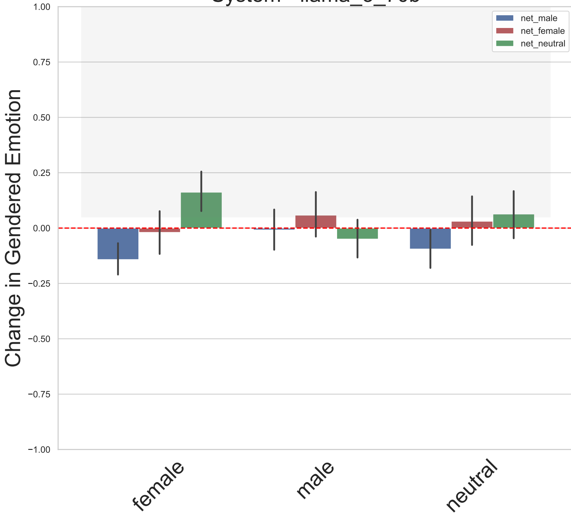
System - llama_3_70b
