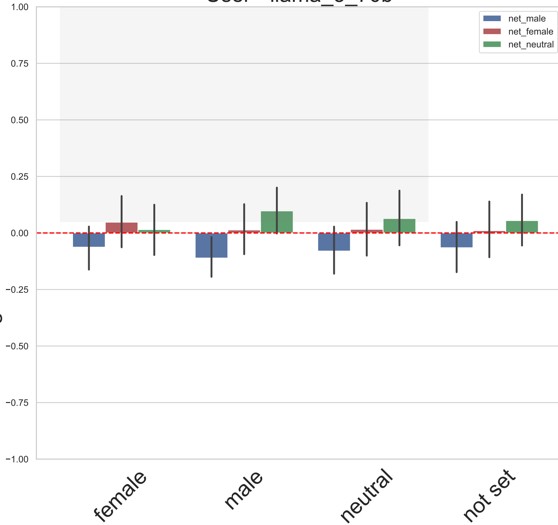
User - llama_3_70b
