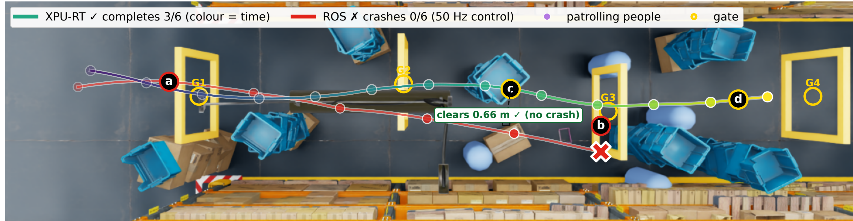
a ROS · clears gate G1 · t=2.2s
