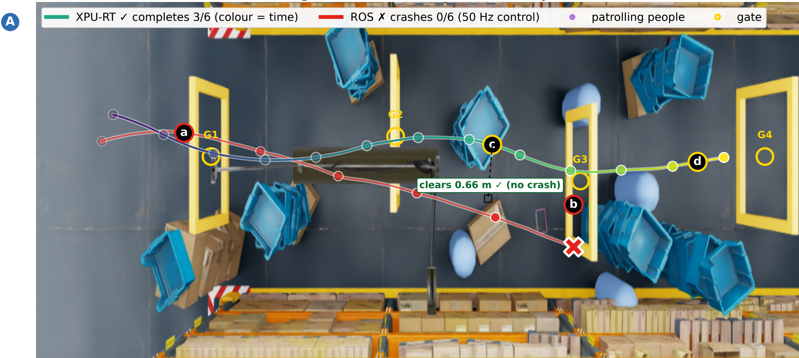
a ROS · clears gate G1 · t=2.2s
