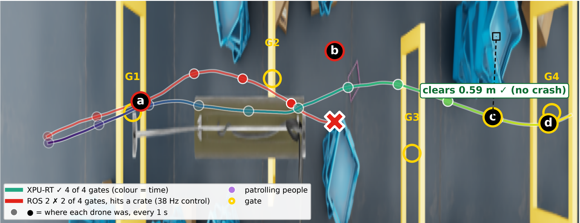
a ROS 2 38 Hz · clears G1 · t=2.8s
