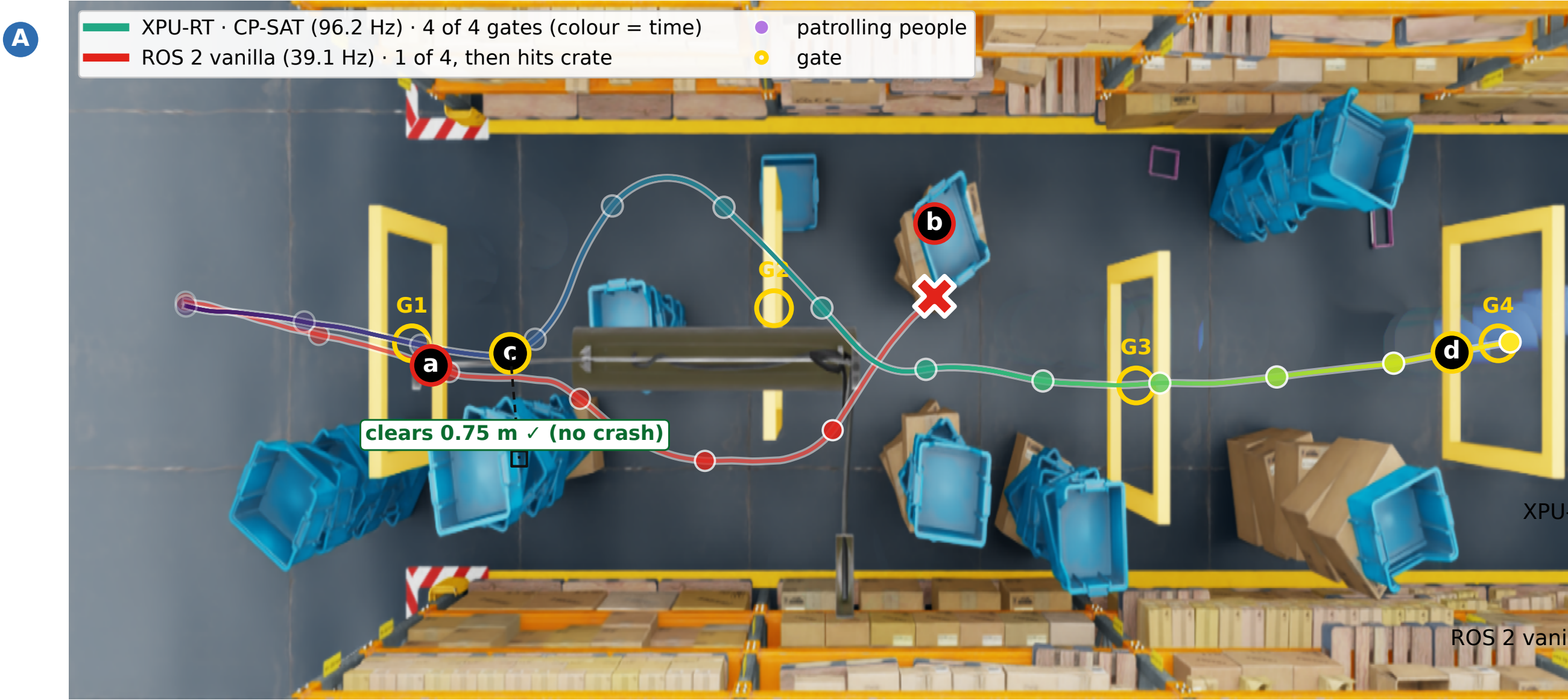
a ROS 2 39 Hz · clears G1 · t=3.5s
