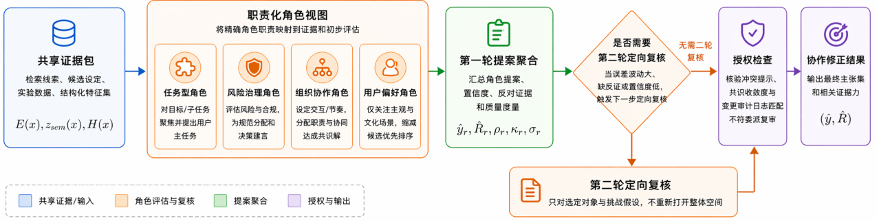
图 2: 职责化协作复核流程。系统先聚合多角色提案，再按需要触发第 2 轮定向复核，并在最终改判前执行授权检查。
