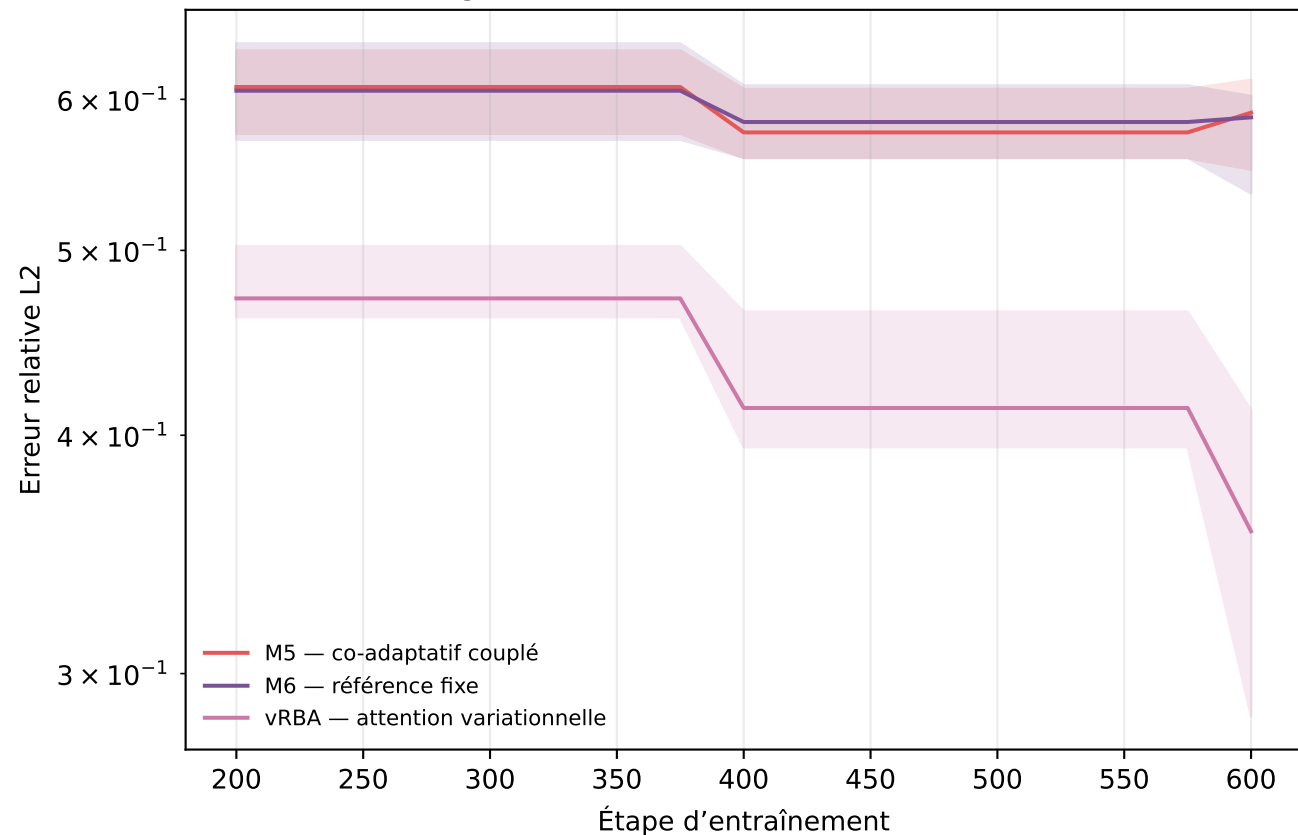
Burgers — vRBA, 13 observations bruitées
