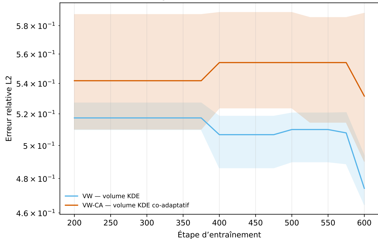
Burgers bruité — KDE 0,5×Scott
