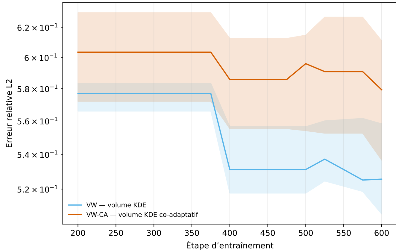
Burgers bruité — KDE 2×Scott
