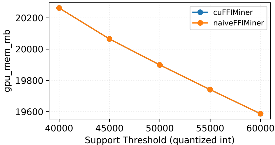
Fuzzy_retail - gpu_mem_mb
