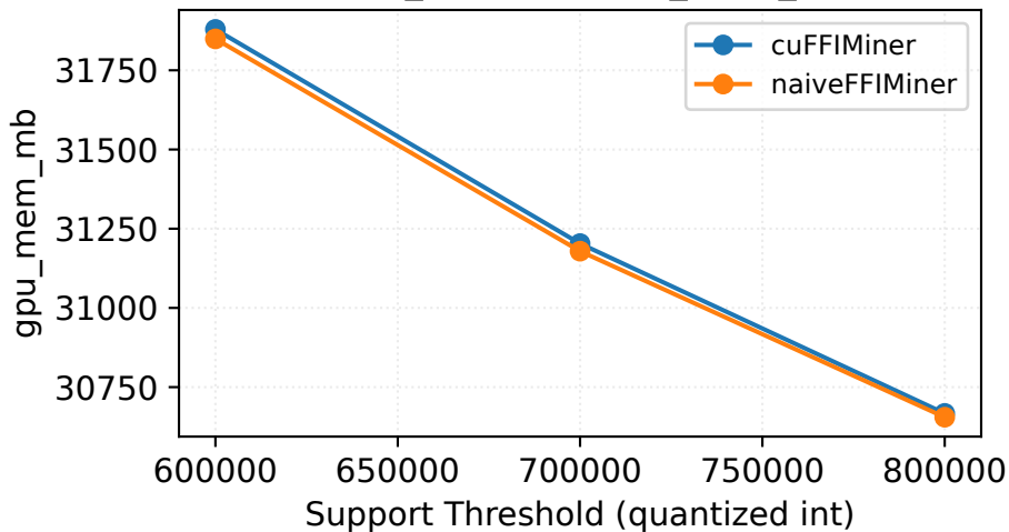
Fuzzy_kosarak - gpu_mem_mb
