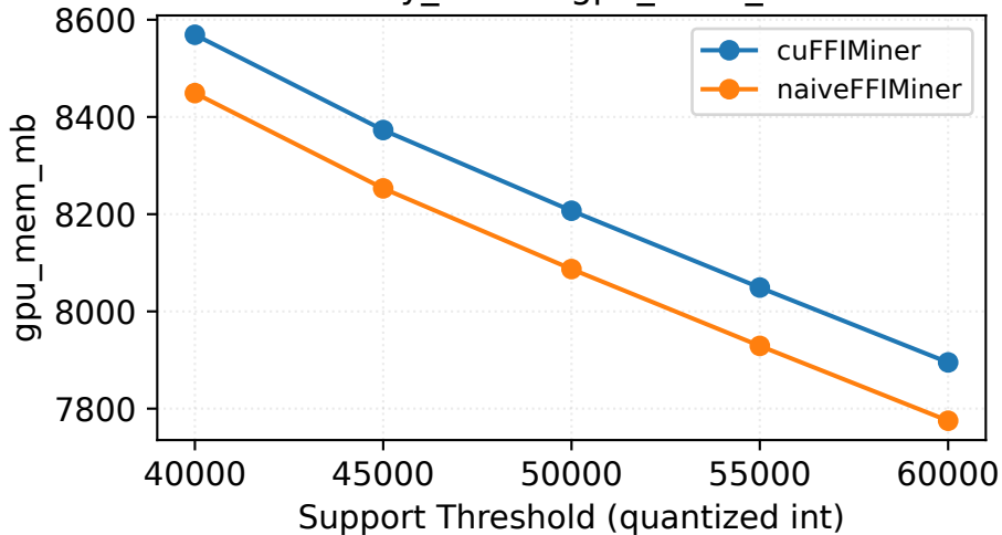
Fuzzy_retail - gpu_mem_mb
