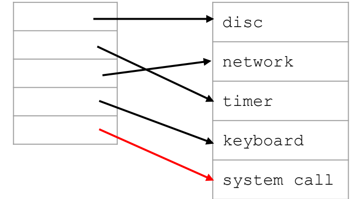
Syscall table
