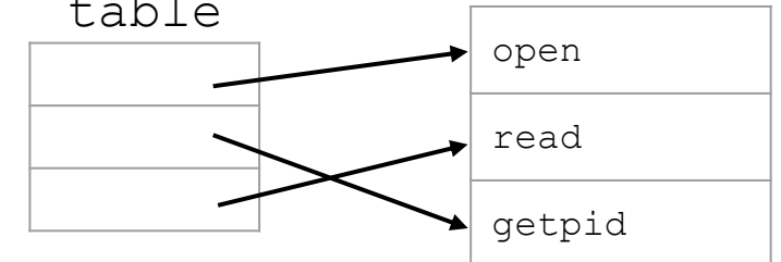
Syscall table
