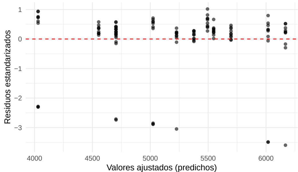
Gráfico de Residuos vs. Valores Ajustados (Homogeneidad de
