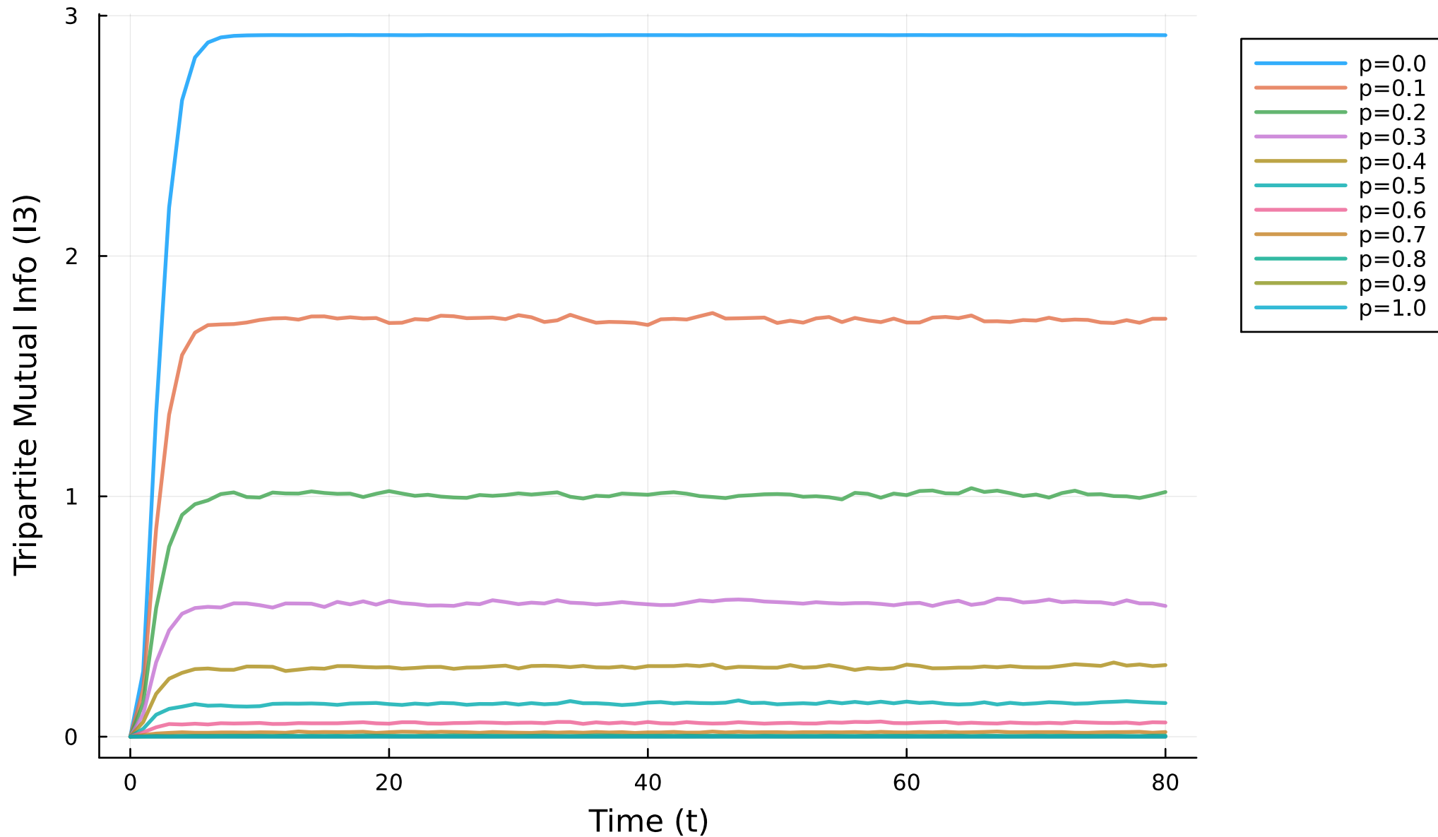
TMI Dynamics (L=8)
