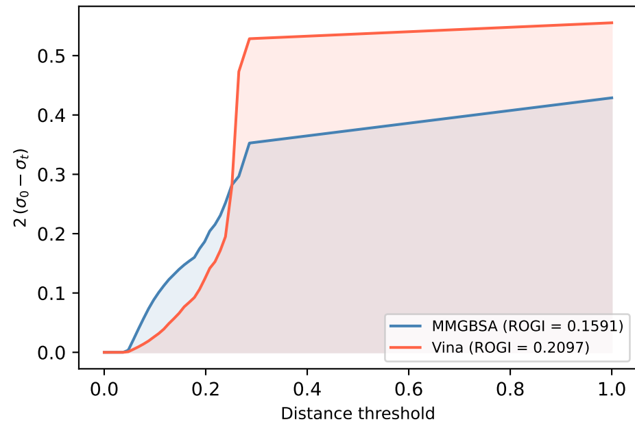
ROGI
