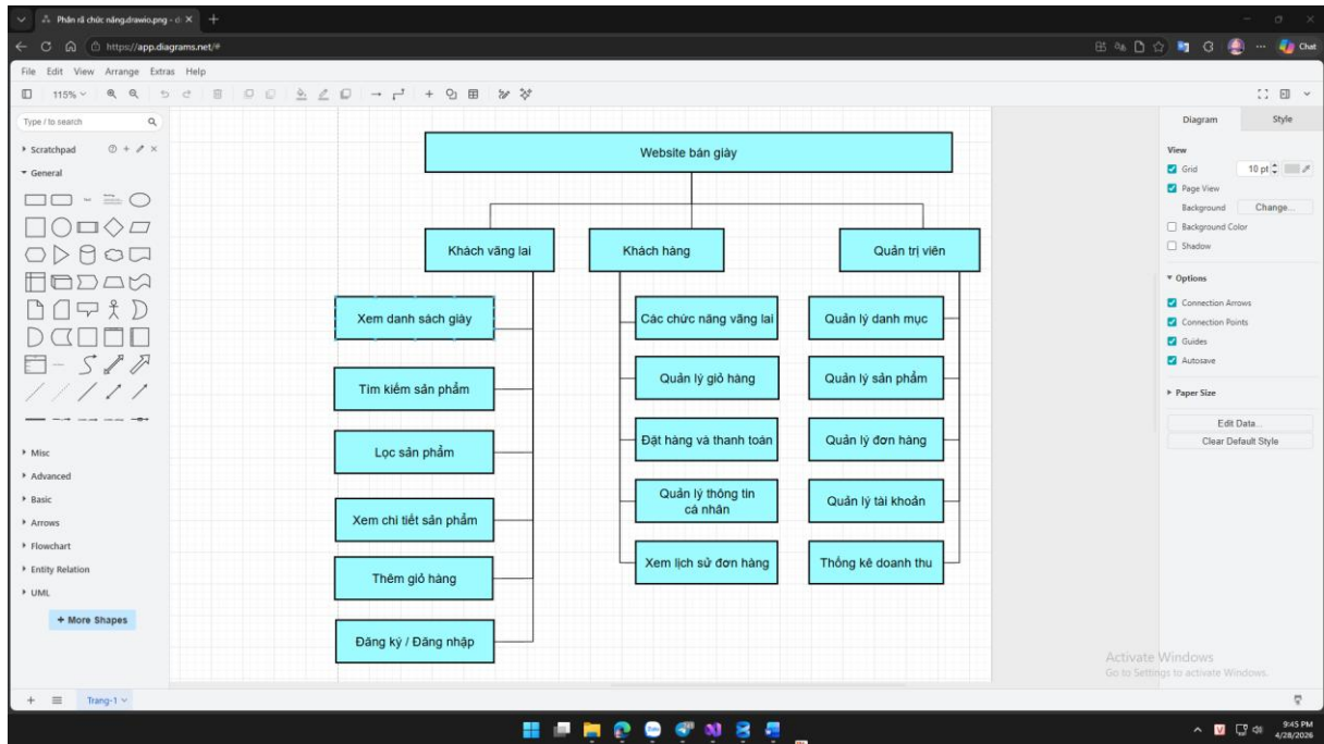
Hình 2. Sơ đồ Phân rã chức năng
