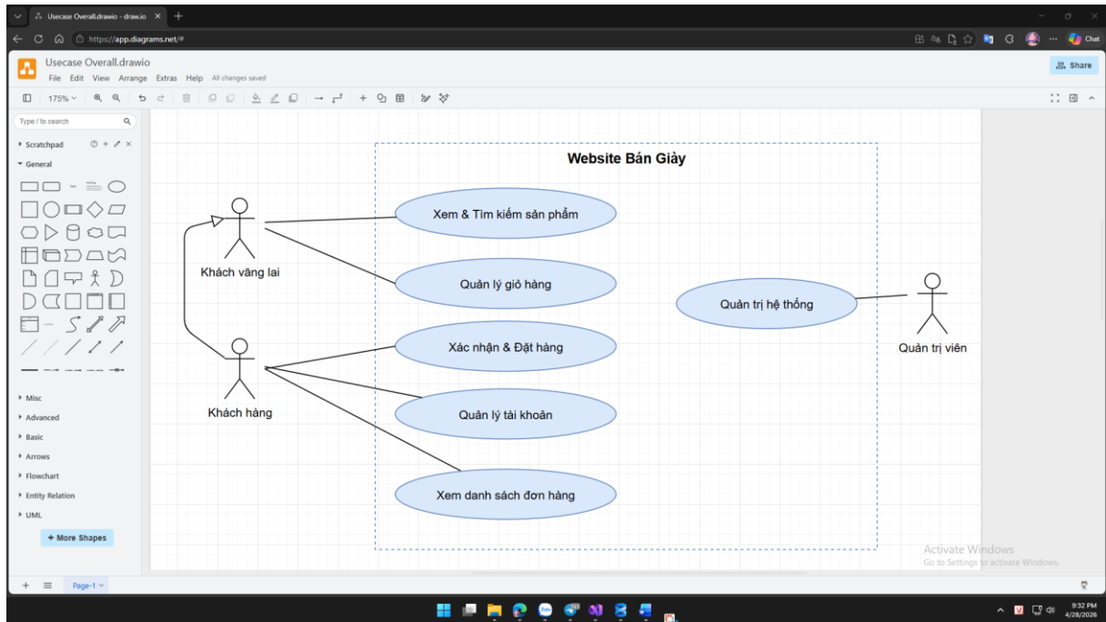
Hình 4. Sơ đồ Usecase Tổng quát
