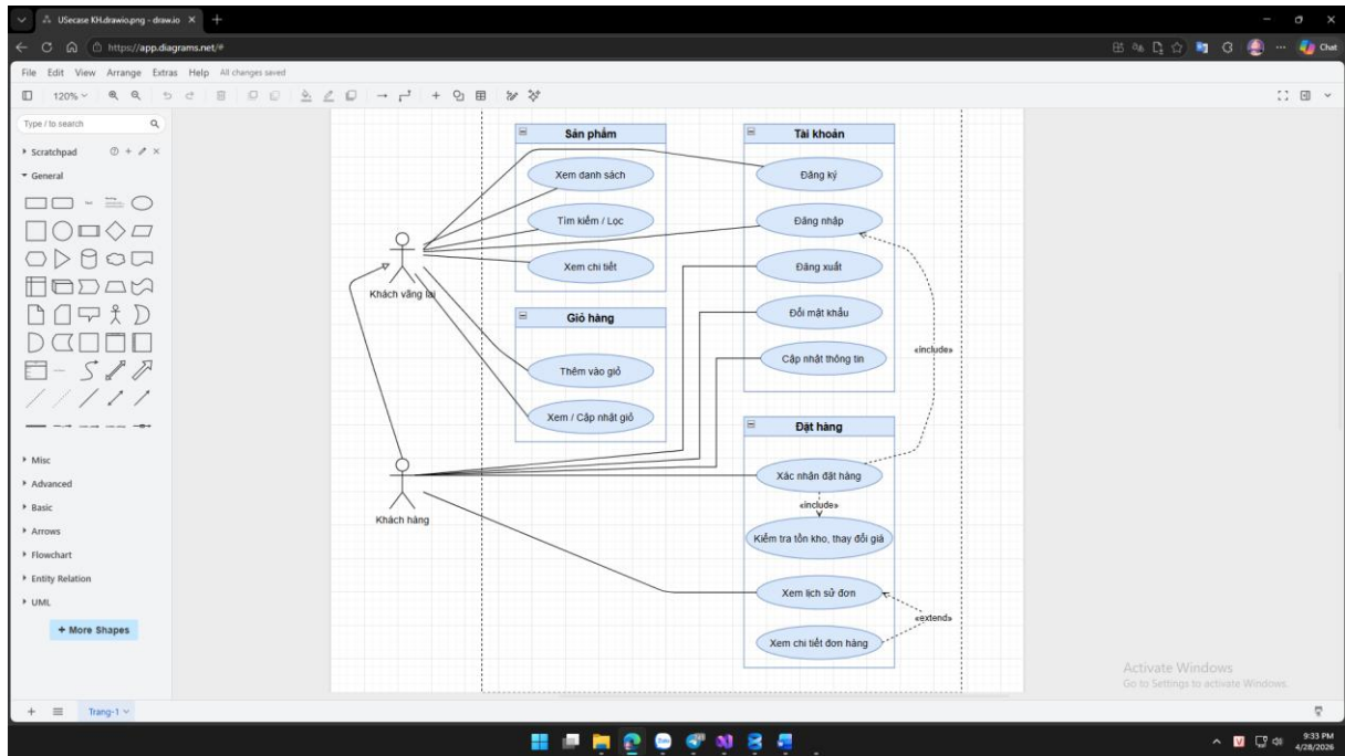
Hình 5. Sơ đồ Usecase của Khách hàng
