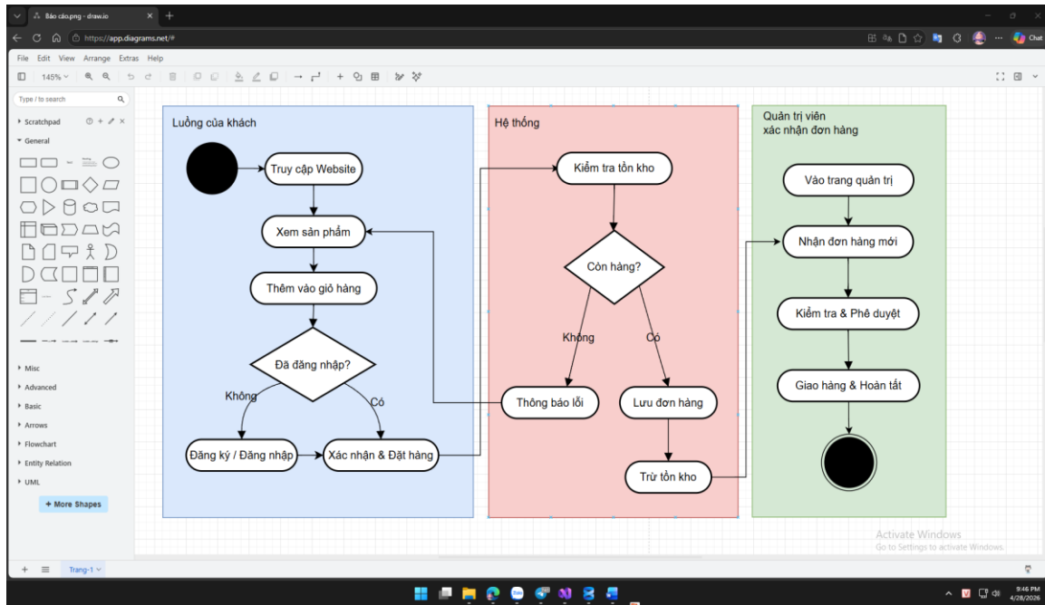
Hình 1. Sơ đồ mô tả bài toán
