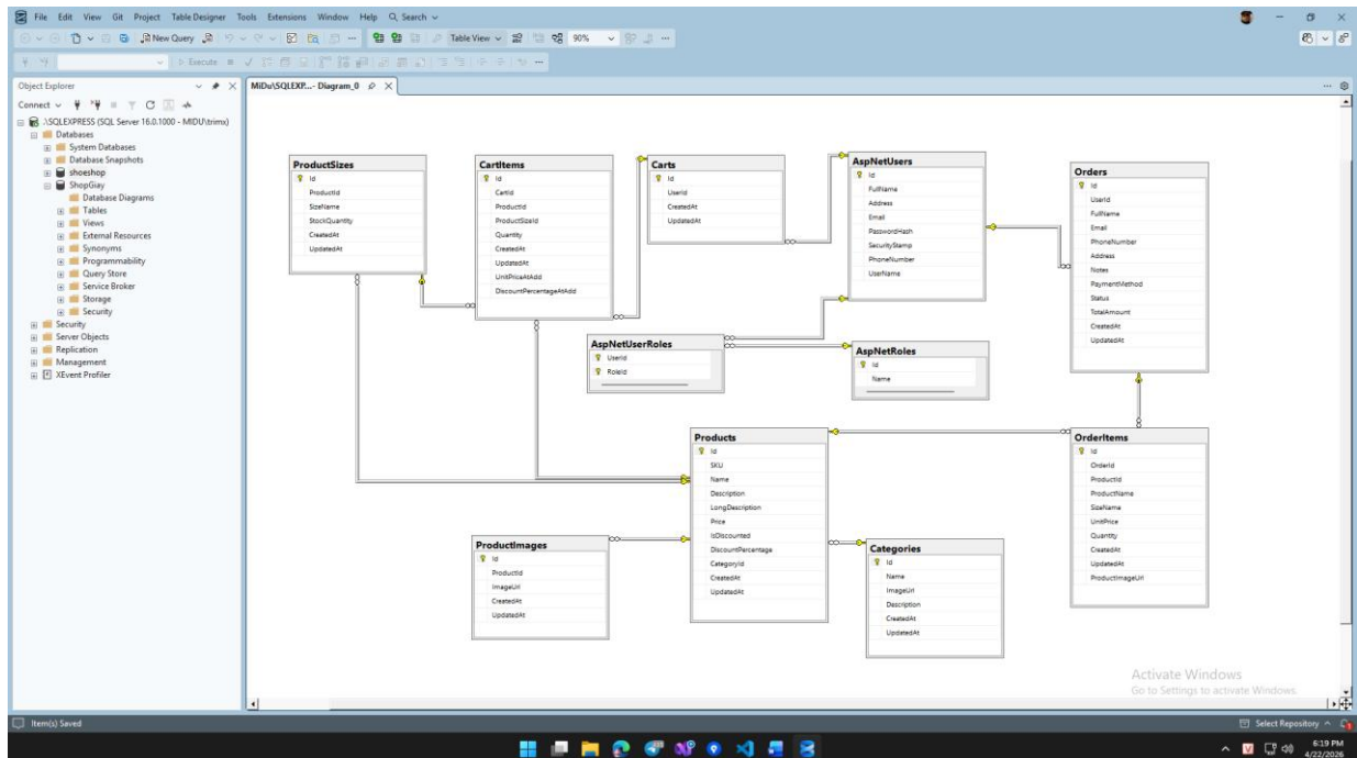
Hình 3. Mô hình dữ liệu quan hệ
