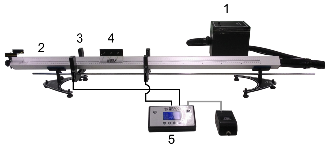
Figura 2: Trilho de ar e acessórios
