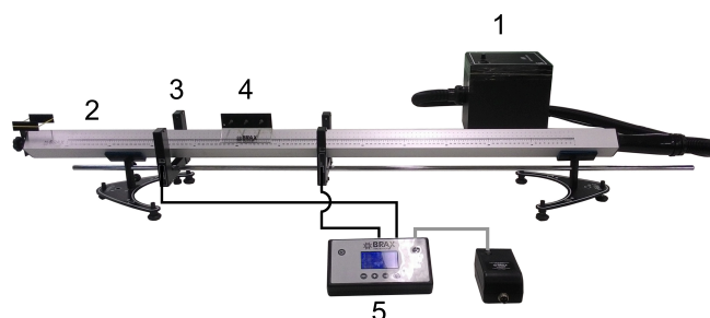
Figura 1: Trilho de ar e acessórios
