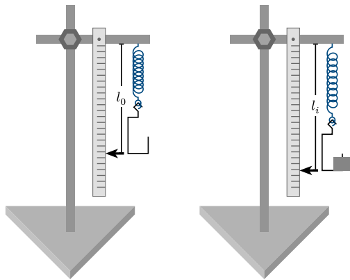
(a) Posição de referência (b) Posição da i -ésima massa
