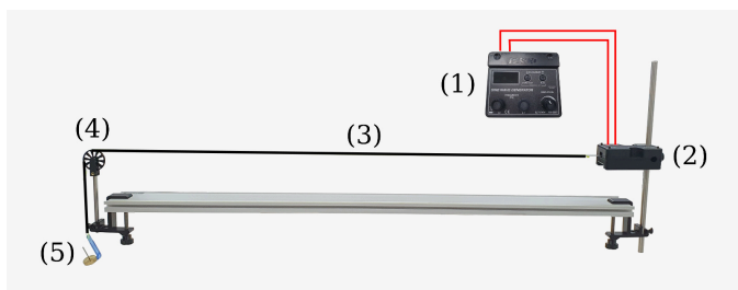
Figura 2: Aparato experimental
