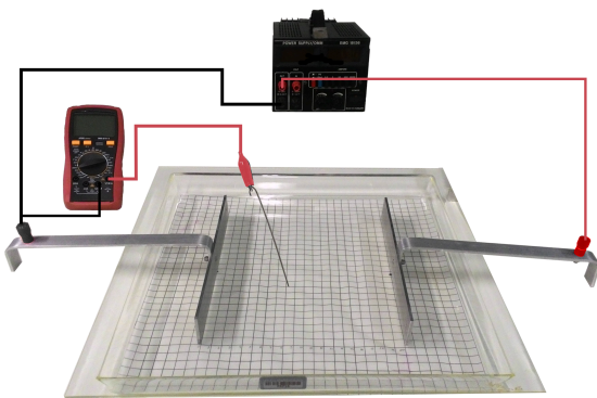
Figura 3: Aparato experimental
