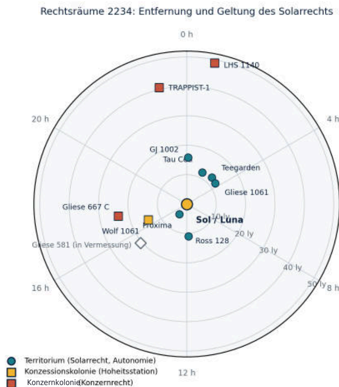
Abb. 1: Rechtsräume 2234 nach Entfernung und Geltung des Solarrechts (Rektaszension und Entfernung).
