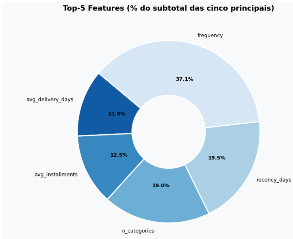
Figura 12 – Top-5 Features por impureza de Gini (Random Forest)
