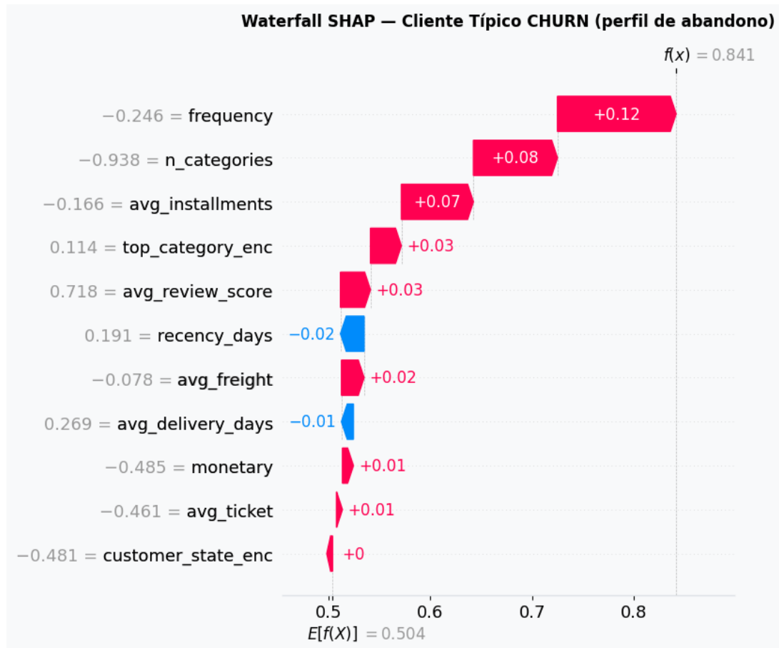
Figura 19 – Decomposição SHAP da predição para o cliente mais próximo do centroide da classe Churn
