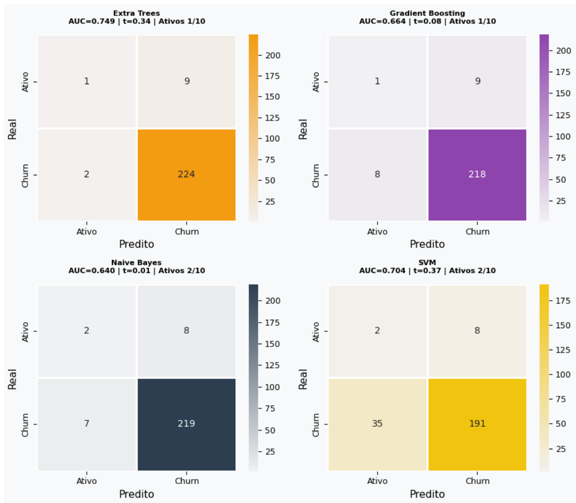
Figura 8 – Matrizes de confusão do Extra Trees, Gradient Boosting, Naive Bayes e SVM no conjunto de teste (limiar out-of-fold)
