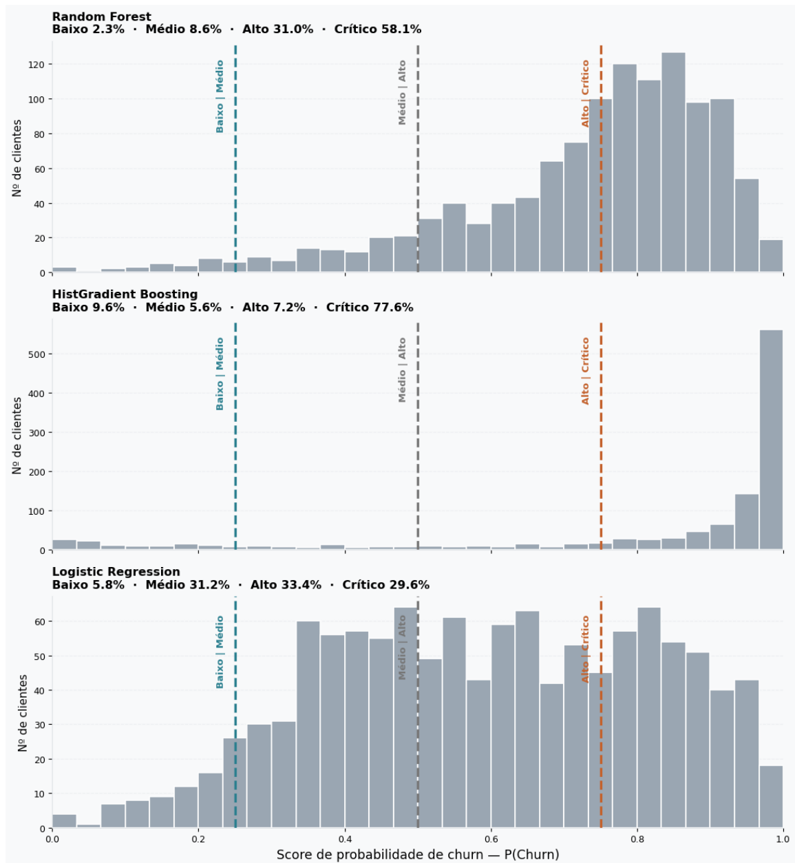
Figura 20 – Distribuição dos scores de probabilidade de churn e limiares de segmentação nos três modelos
