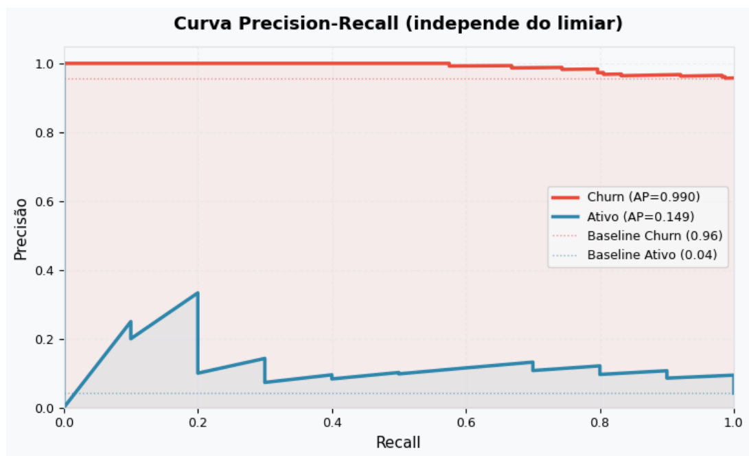
Figura 10 – Curva Precision-Recall por classe, independente do limiar (Random Forest)
