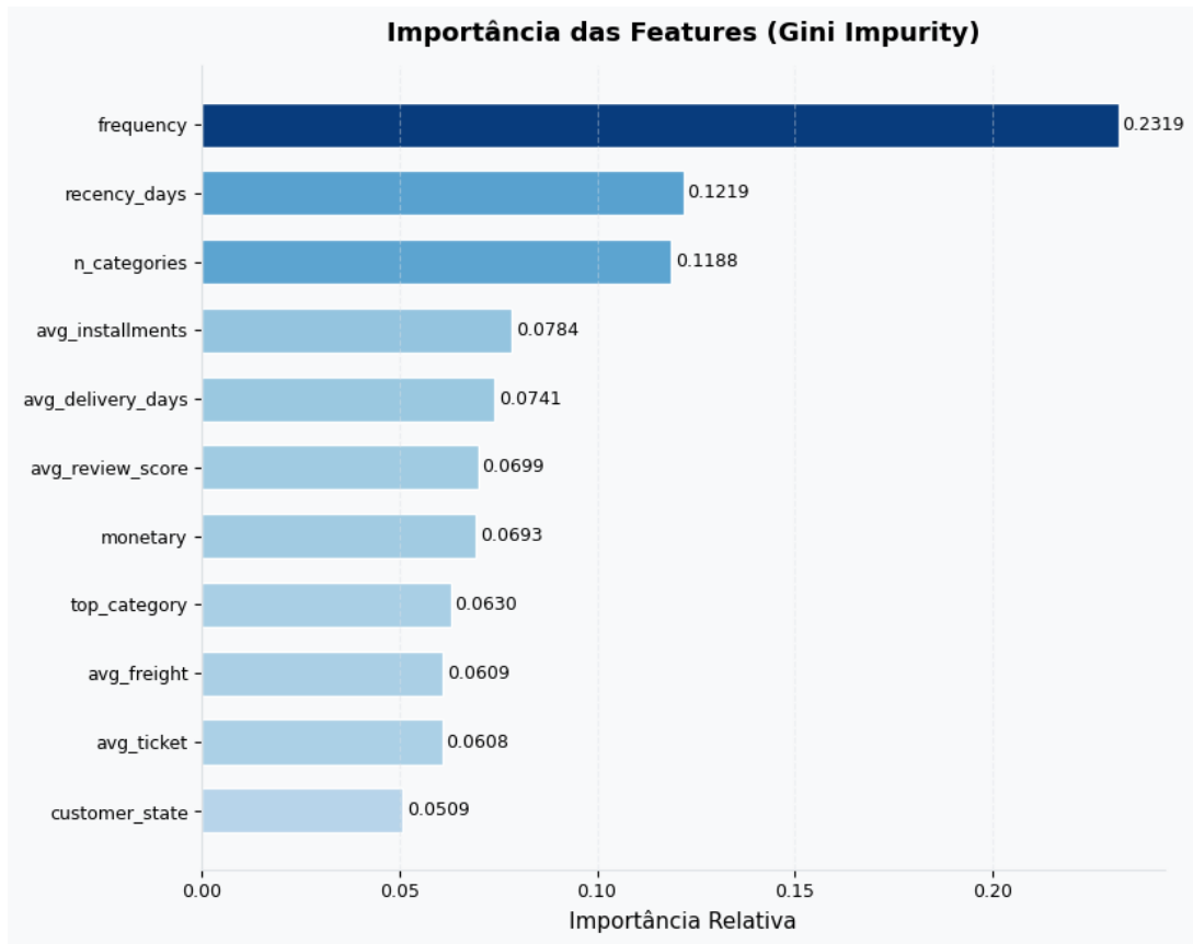
Figura 11 – Importância das features por impureza de Gini (Random Forest)
