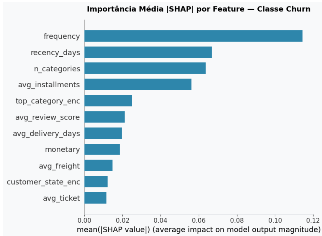
Figura 13 – Importância média |SHAP| das features (Random Forest)
