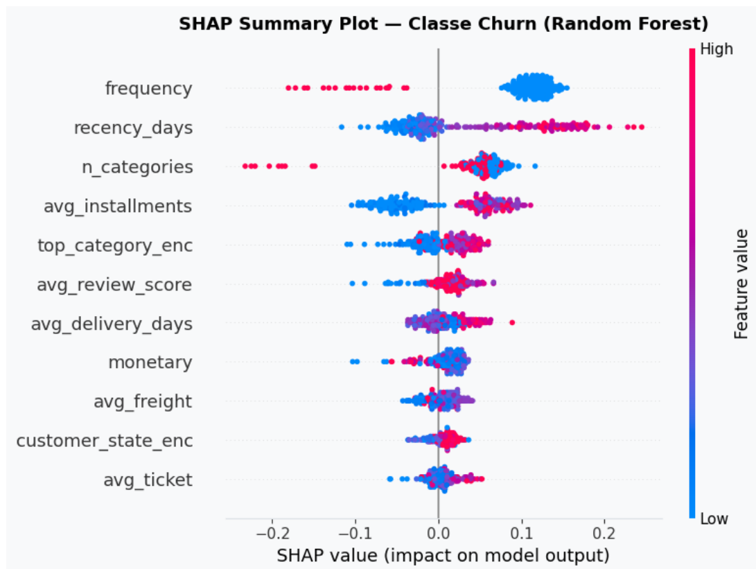
Figura 14 – Valores SHAP (beeswarm) das features no conjunto de teste
