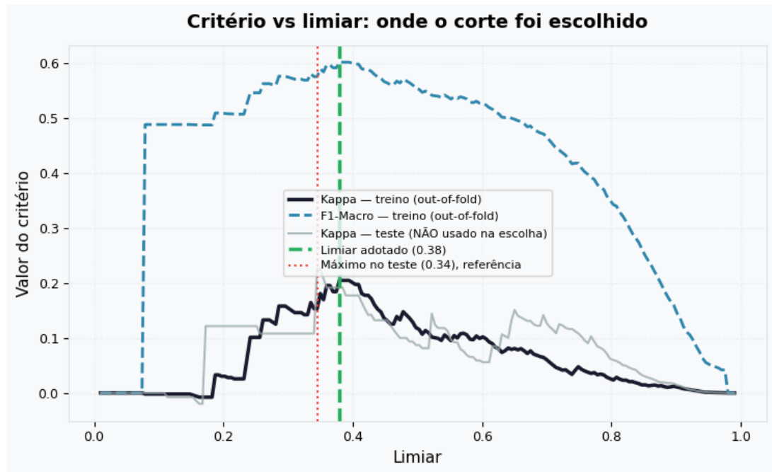
Figura 9 – Critério de escolha do ponto de corte em função do limiar (Random Forest)
