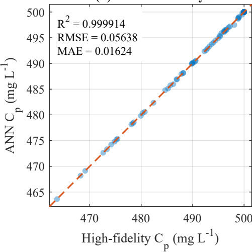
(d) Product salinity
