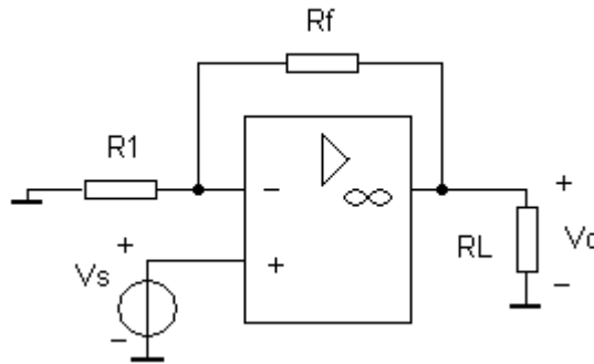
图 4-3 同相放大器
