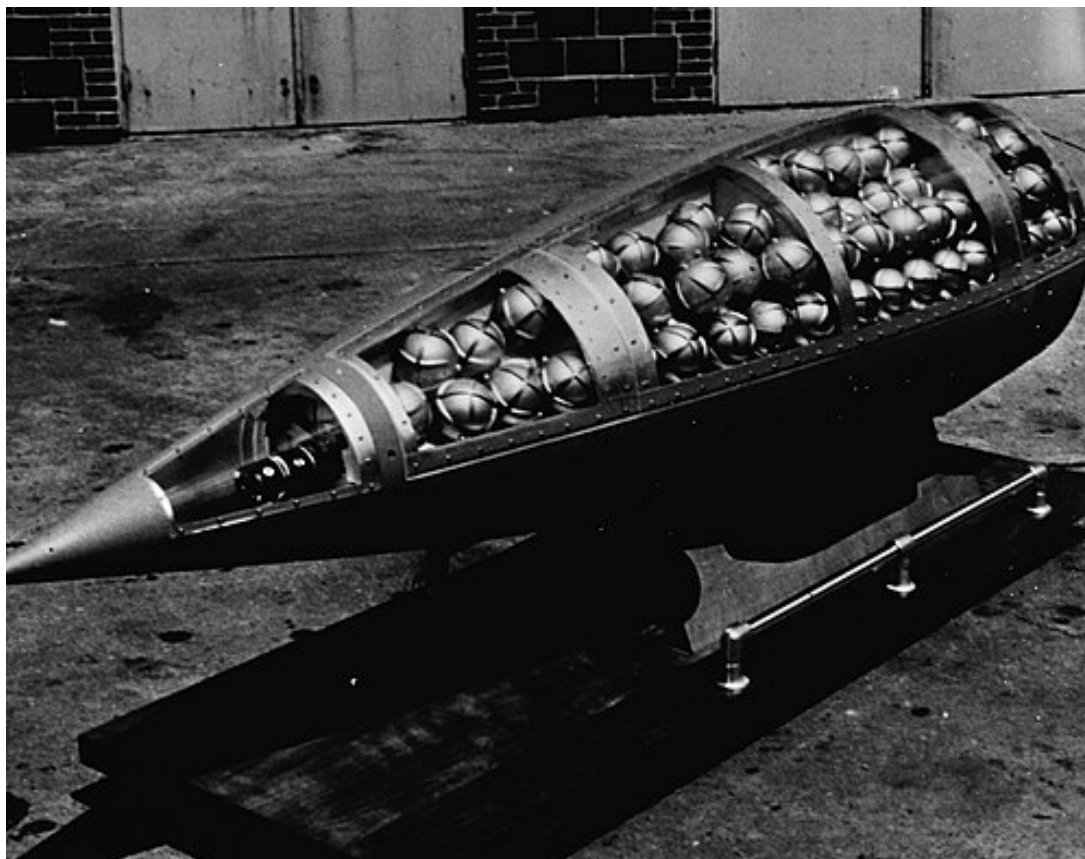
Rysunek 110: KPOM-2 – kasetowy element minowy
