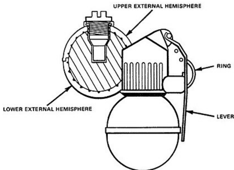
Rysunek 96: RGN – granat ofensywny z zapalnikiem uderzeniowym
