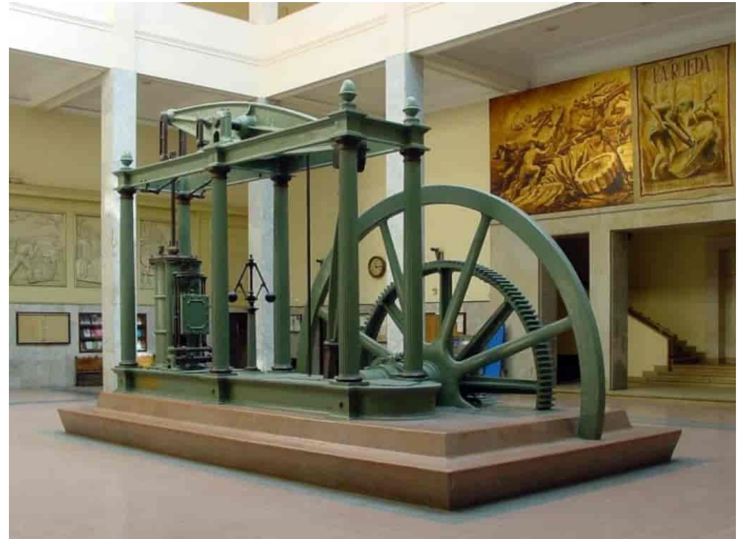
Dampmaskin
