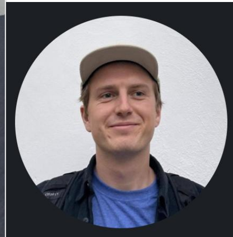
Peder Hognestad
