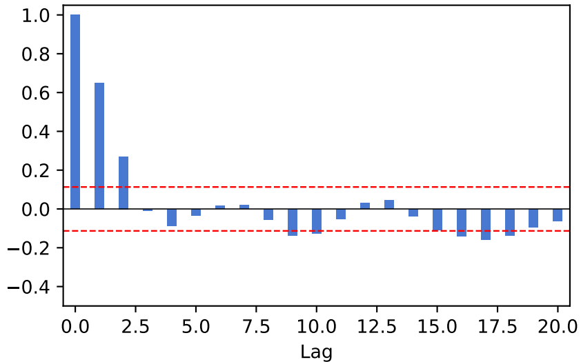
MA(2) — ACF
