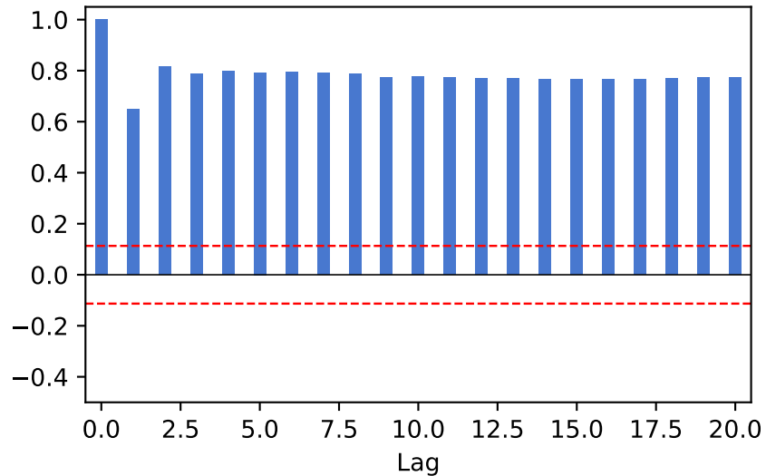
MA(2) — PACF
