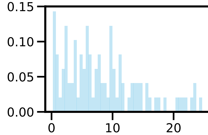
R/L_{T_i}
