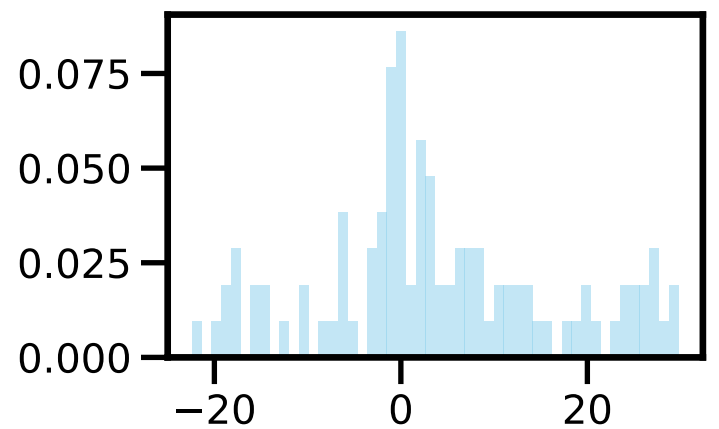
pfi_gb
