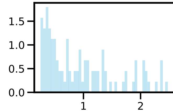
\log_{10} \nu_{ee}
