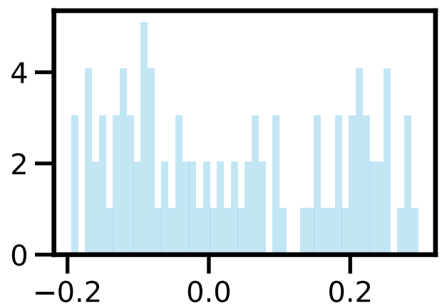
pfi_gb
