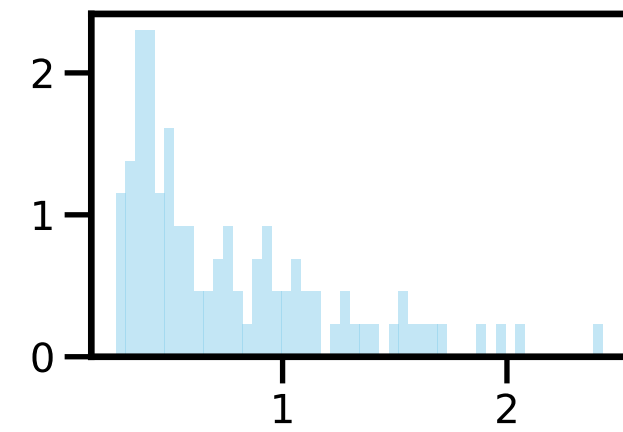
\log_{10} \nu_{ee}
