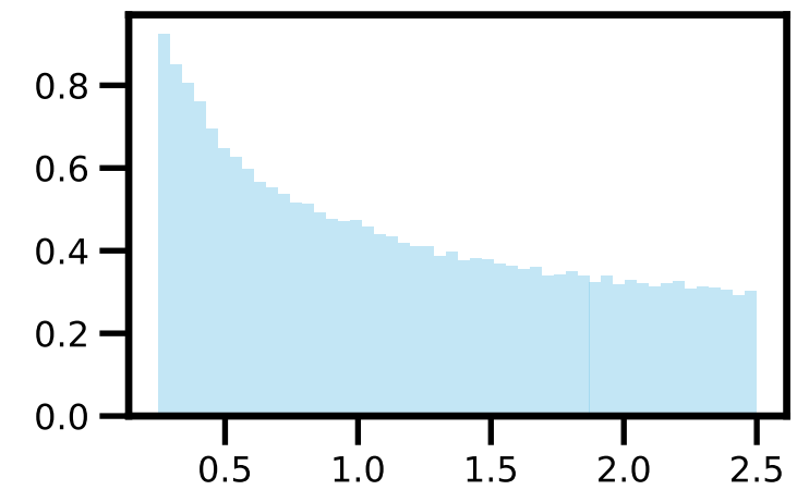
\hat{s}
