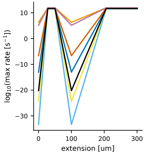
Peierls
