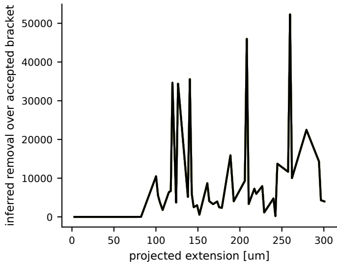
discard/escape accounting
