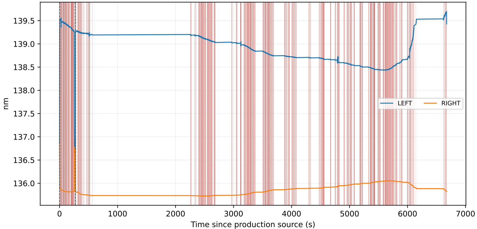
Contact radii
