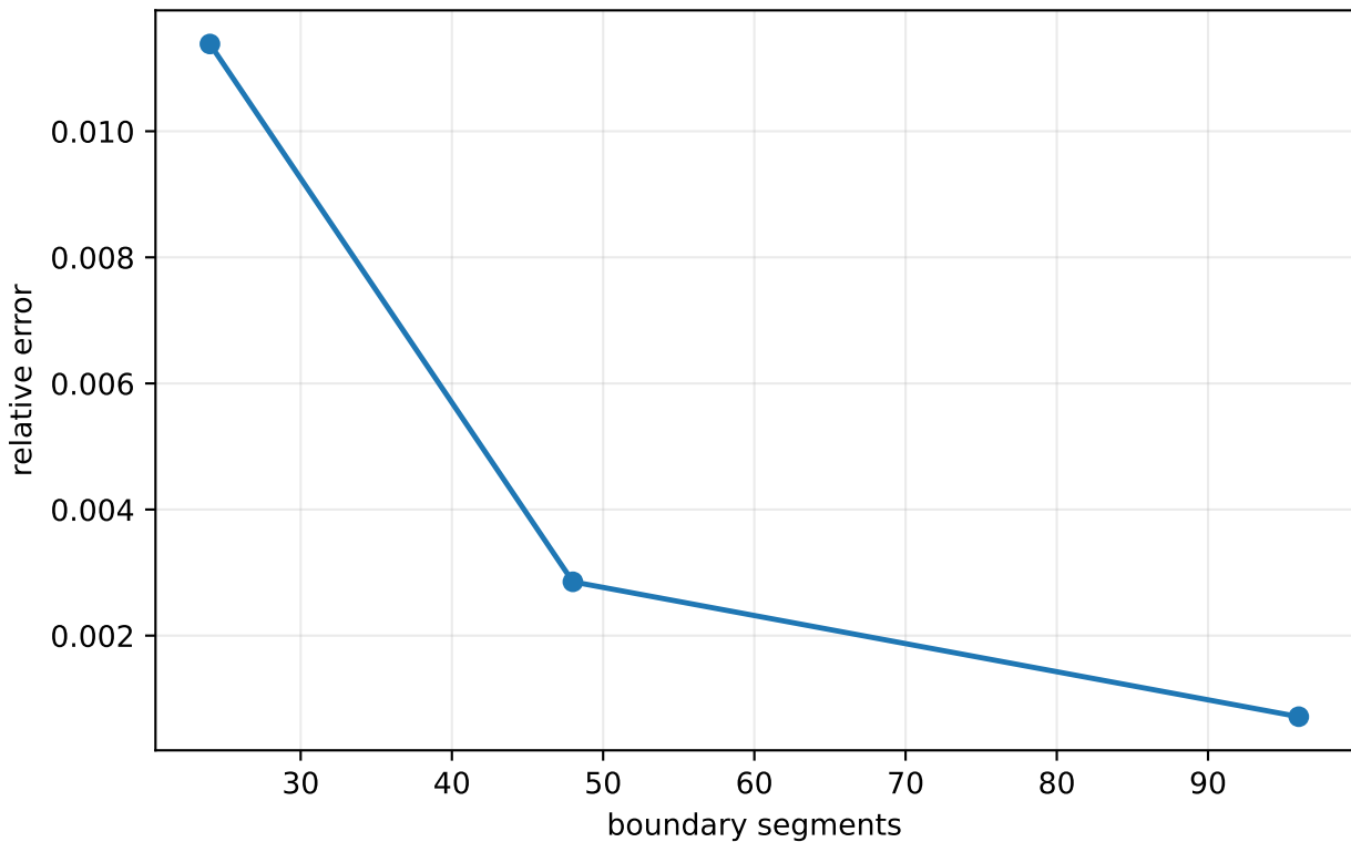
VOIDING V1 CRACK VOID MESH CONVERGENCE
