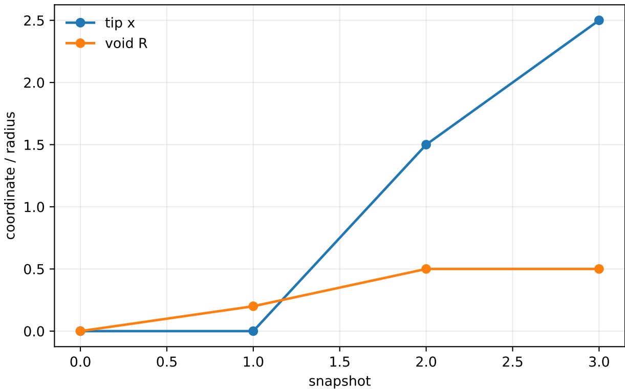
VOIDING V1 ONE VOID GEOMETRY SNAPSHOTS
