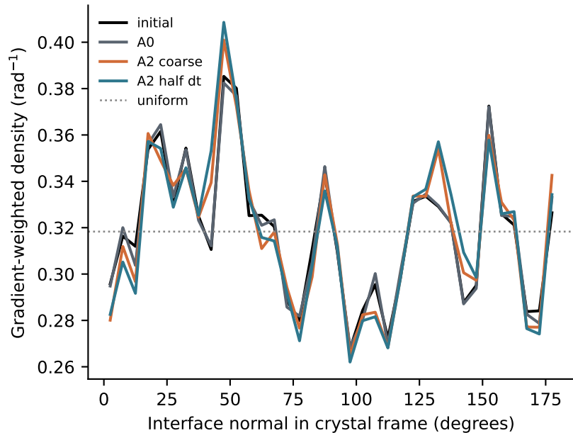
Crystal-frame interface normals
