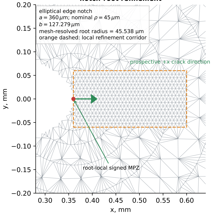
notch-root refinement
