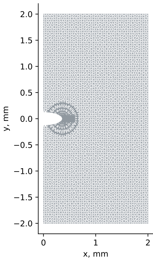
actual K360 elastic FEM mesh
