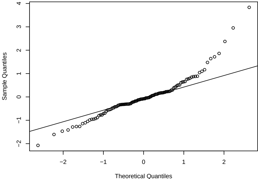
CO2 – normal Q-Q
