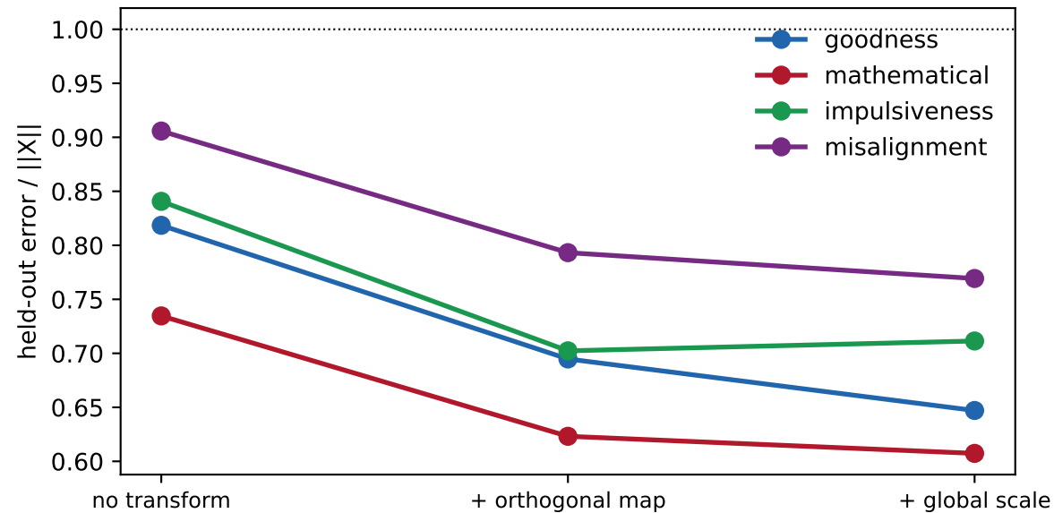
CV: hold-out traits
