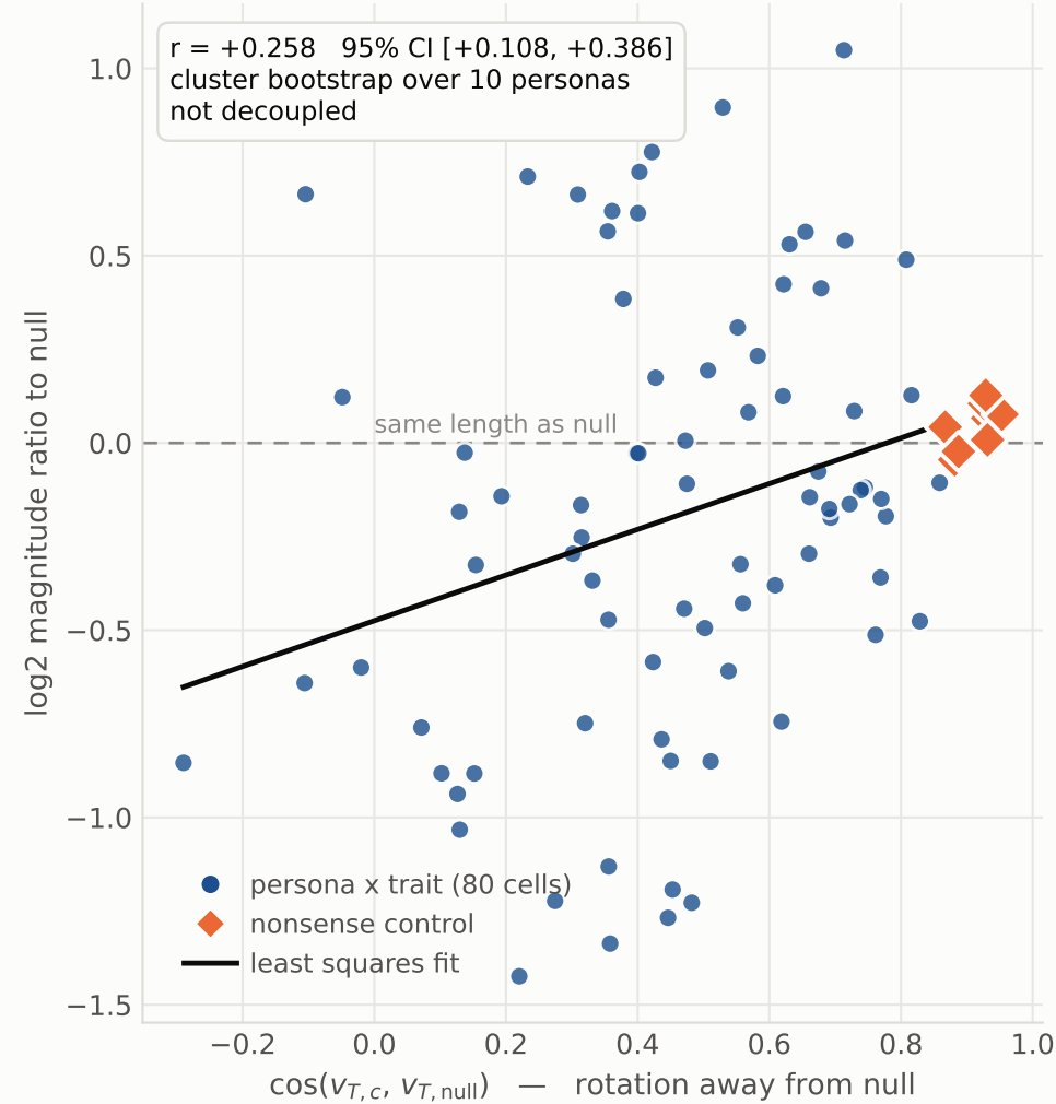
B. B.6 decoupling test, layer 25
