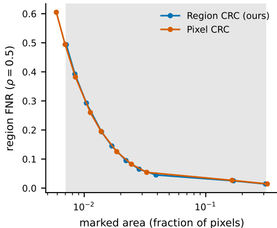
SegFormer-B5
