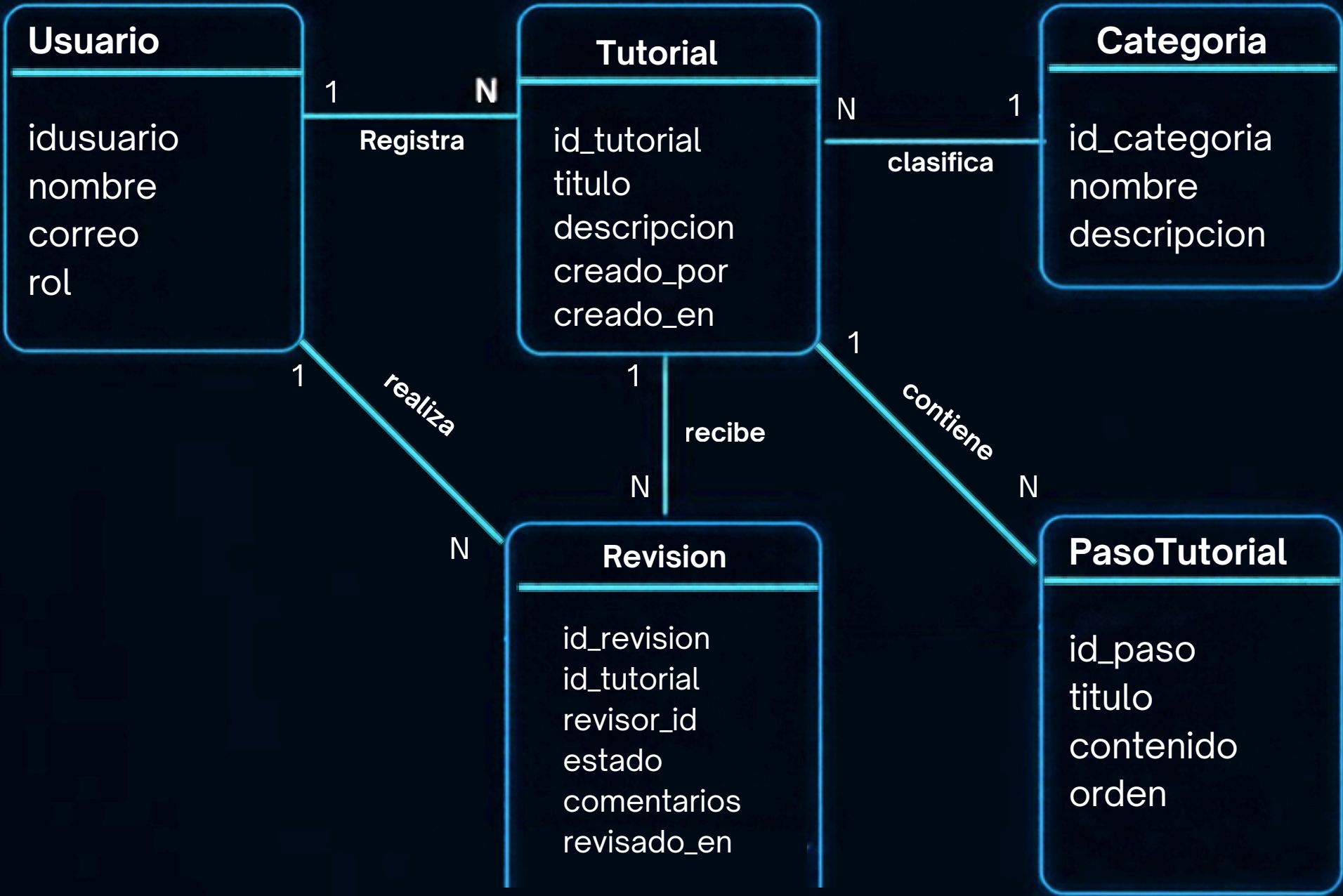
MODELO DE DATOS
