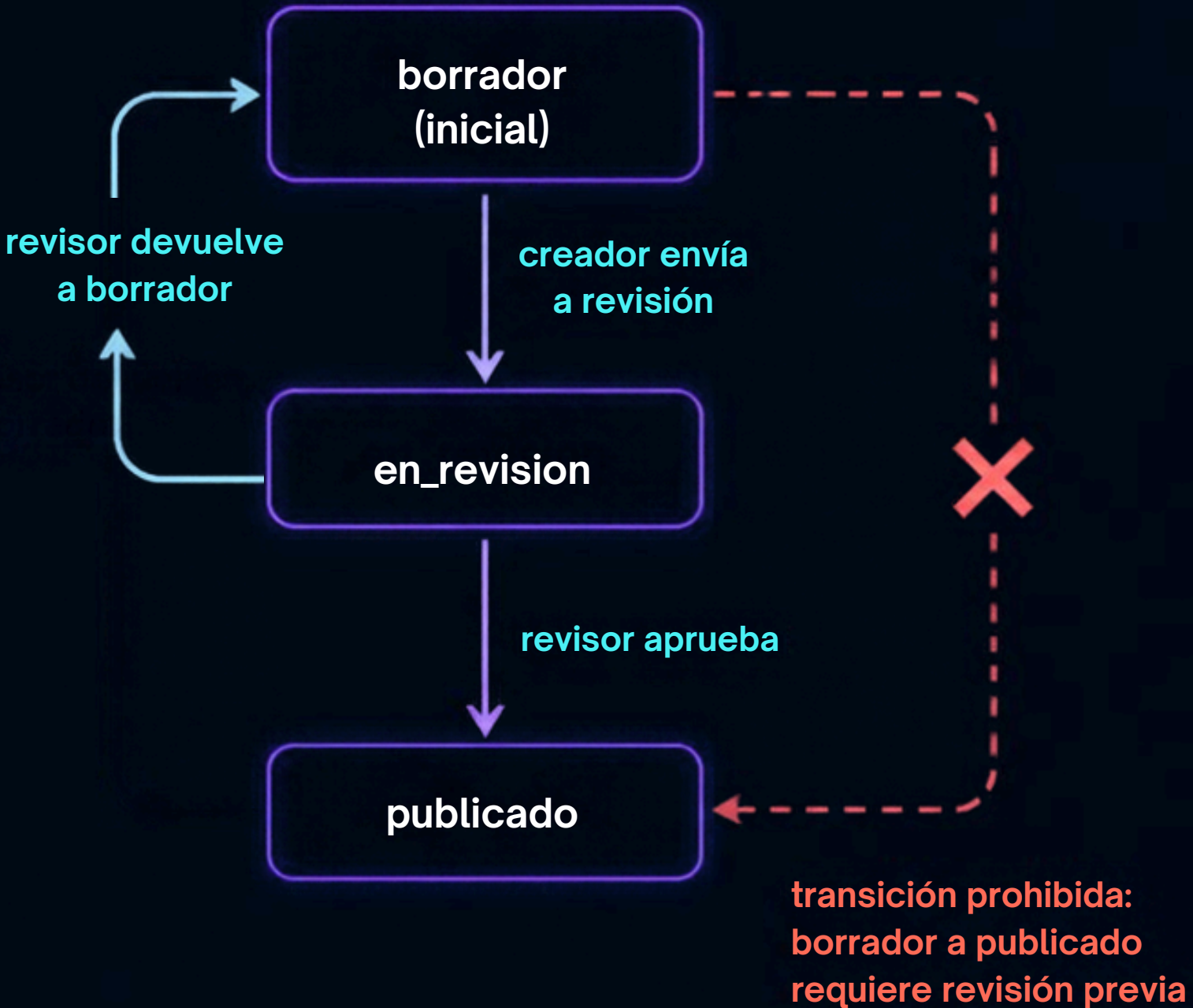
MÁQUINA DE ESTADOS DEL TUTORIAL
